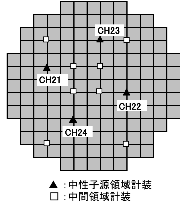
島根2号機炉心配置
