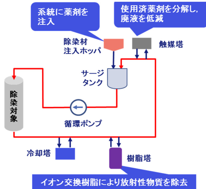
系統除染の例(化学的除染の場合)
