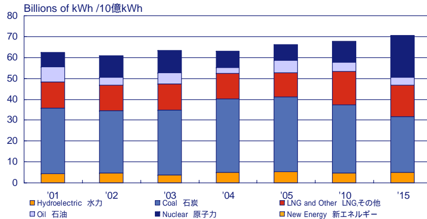
電源種別発電電力量
