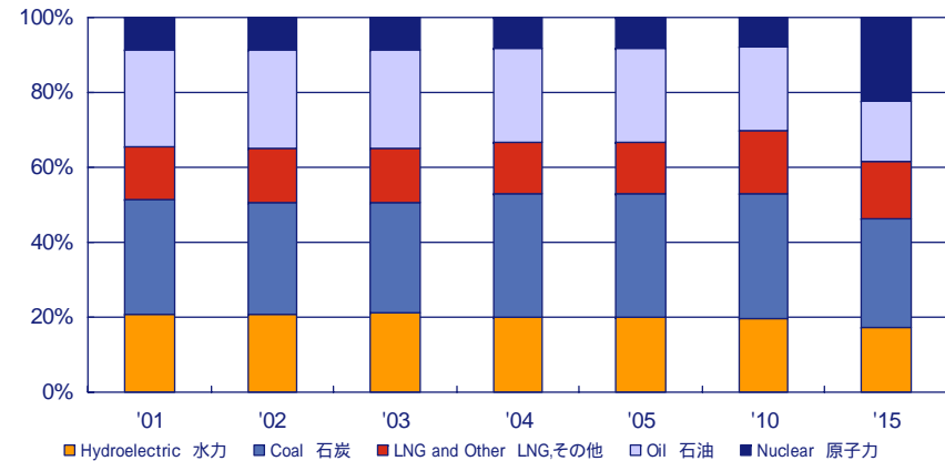
電源種別発電設備構成比
