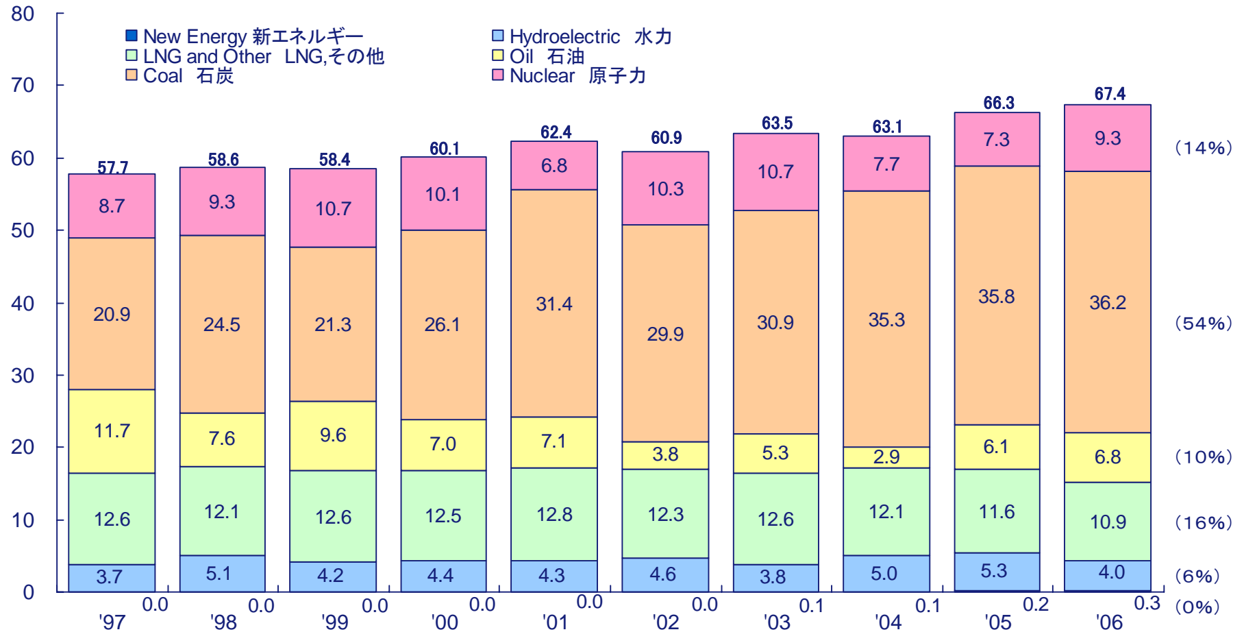
The Power Generation by Type 電源種別発電電力量 (Billions of kWh/10億kWh)
