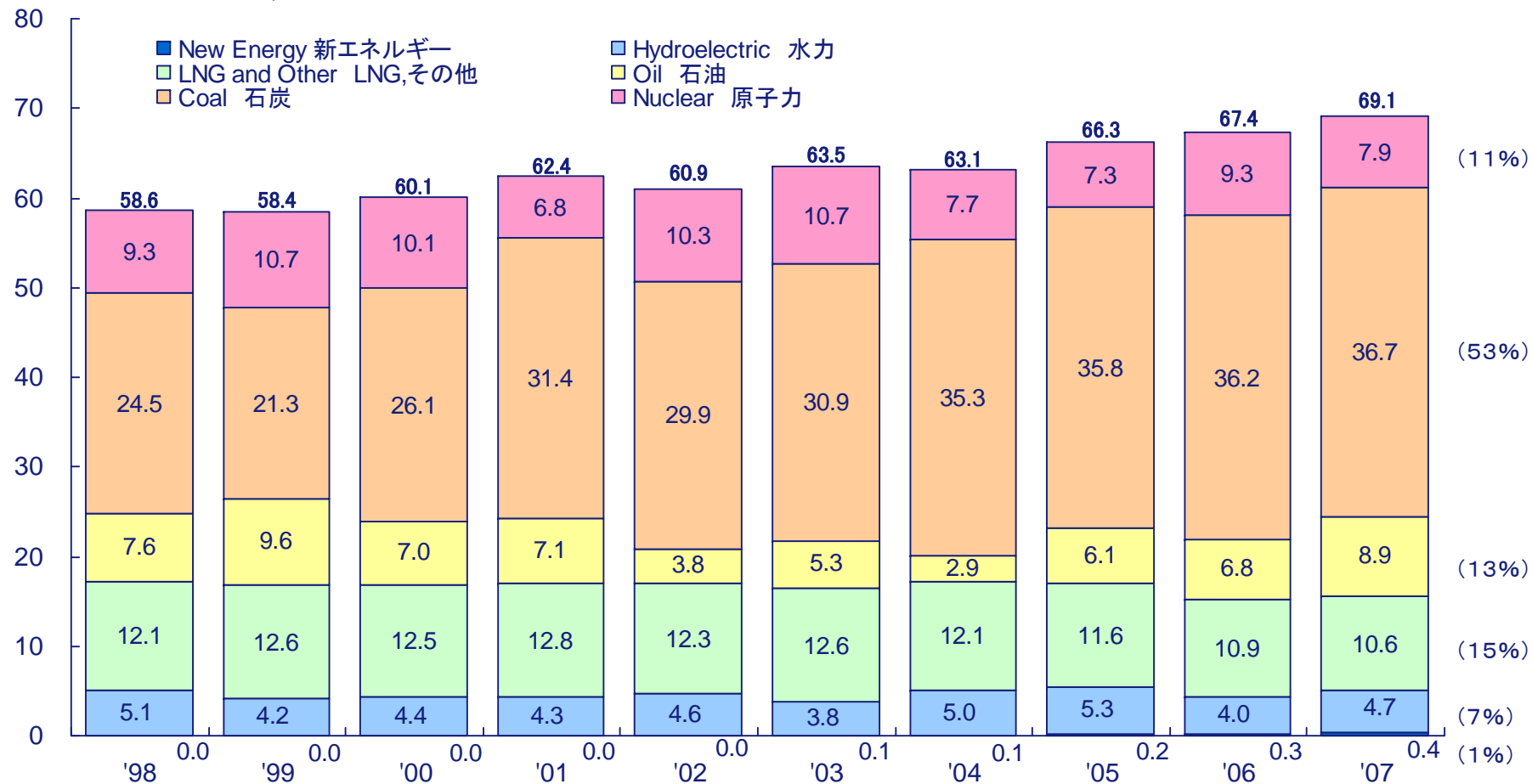
The Power Generation by Type 電源種別発電電力量 (Billions of kWh/10億kWh)
