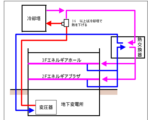
排熱利用設備
