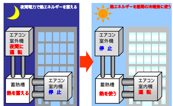
蓄熱式空調の概要
