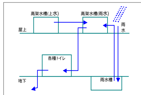
雨水の利用設備
