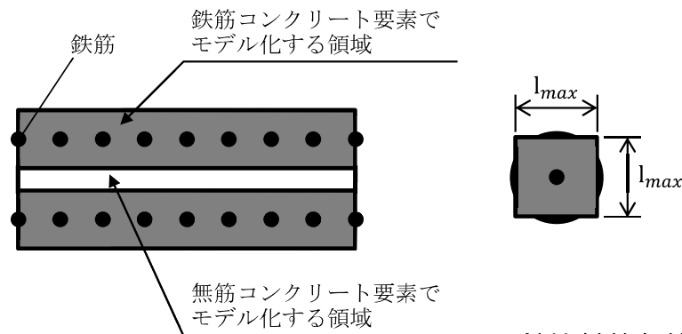
鉄筋付着有効領域と無筋領域の分割の概要
