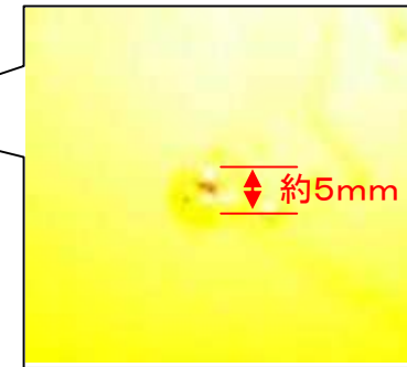
▲腐食部(貫通孔)拡大写真
