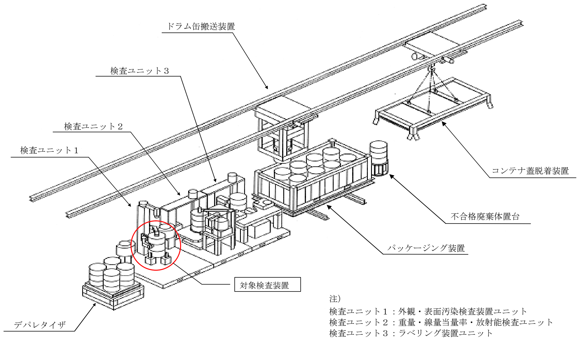
低レベル放射性廃棄物検査装置鳥瞰図
