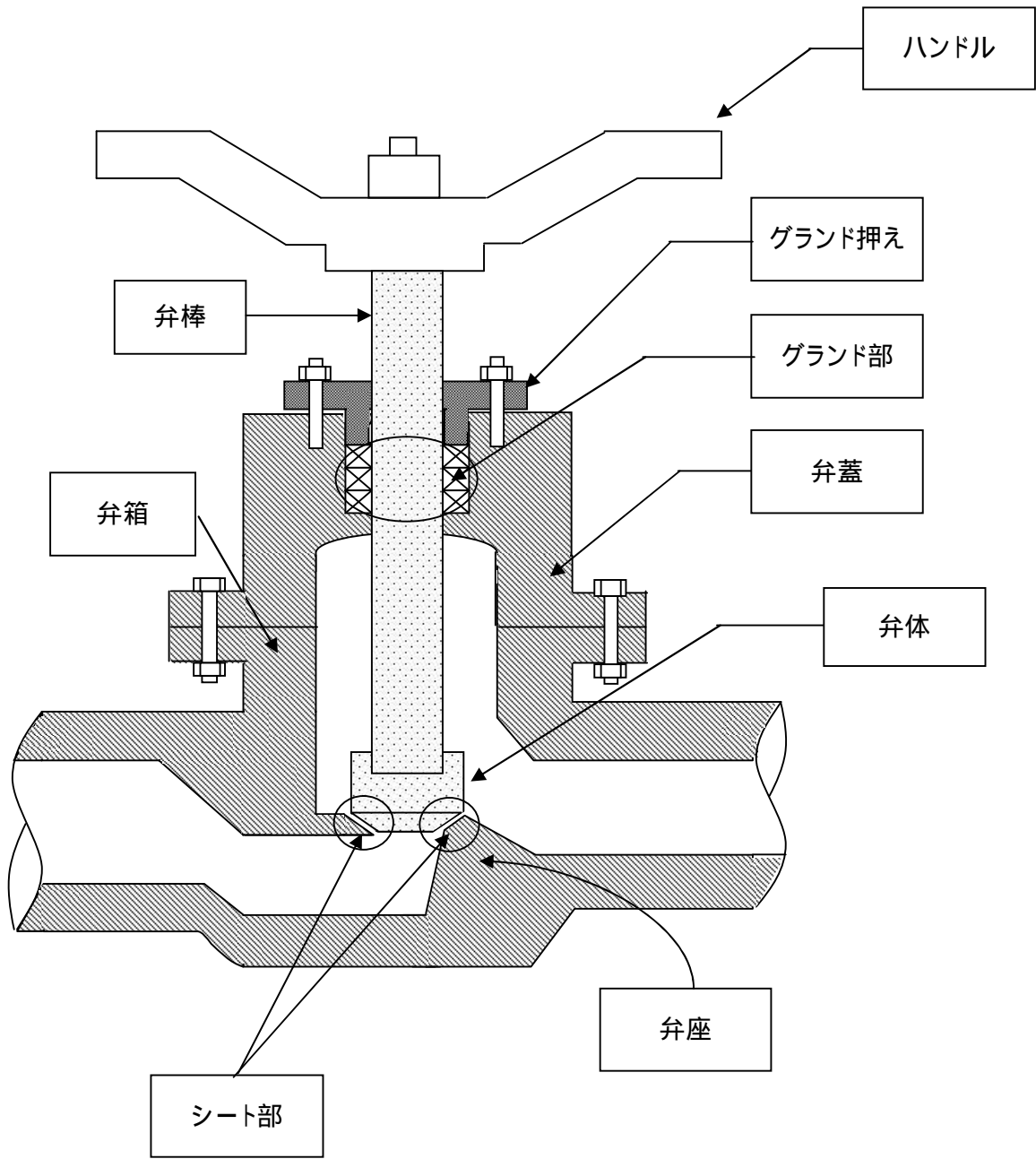
弁構造図
