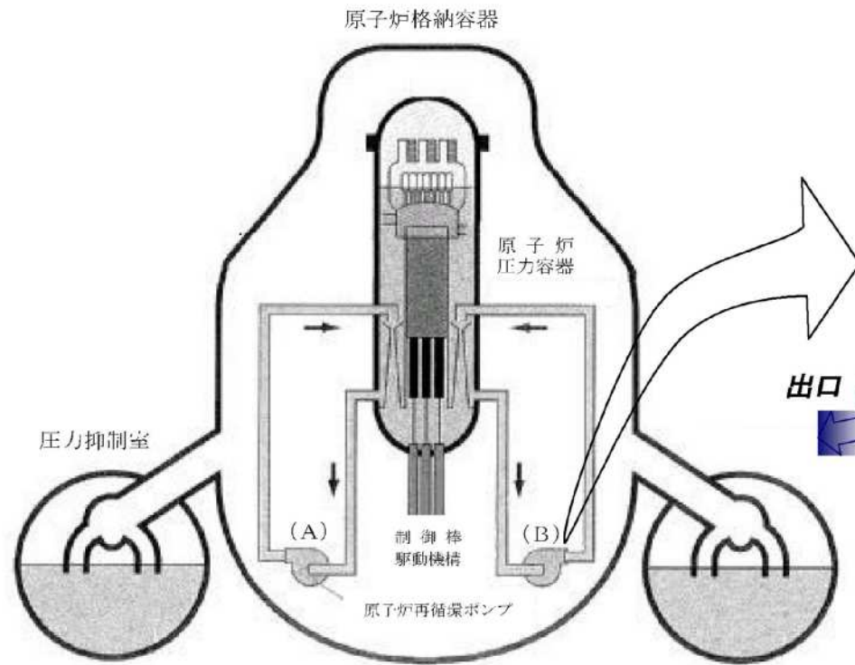
原子炉格納容器内概略
