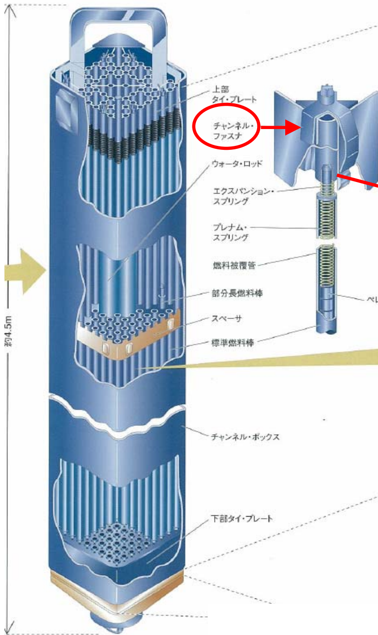
燃料集合体
