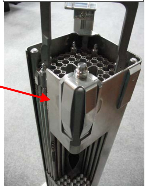
【燃料集合体(模型)】
