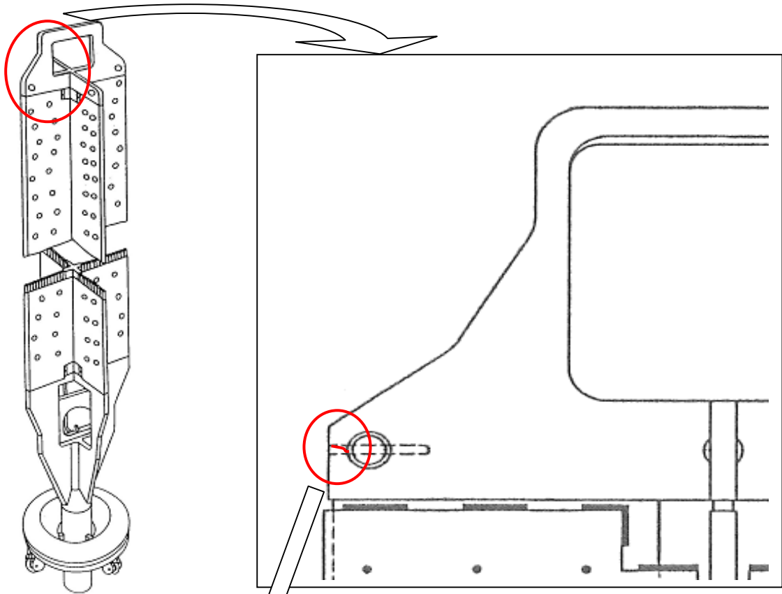
制御棒外観全体図
