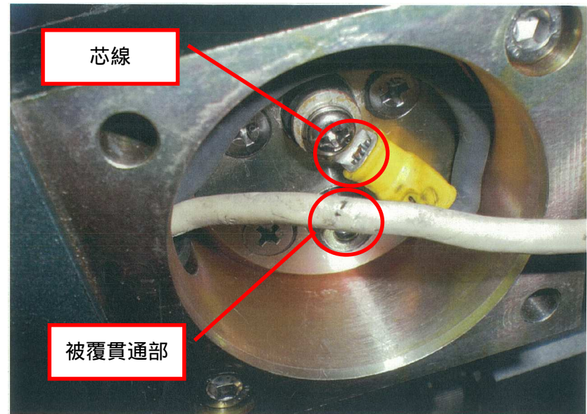
継電器盤および電磁弁電源端子箱内の状況
