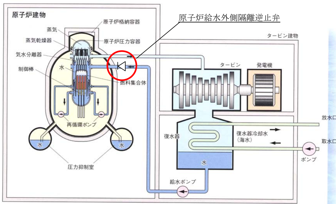
原子炉給水外側隔離逆止弁位置図
