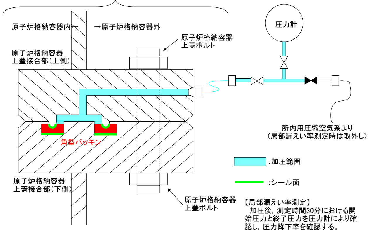
原子炉格納容器上蓋部の局部漏えい率測定 概要図
