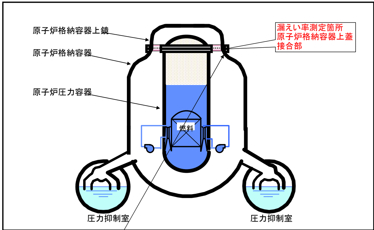
原子炉格納容器概要図
