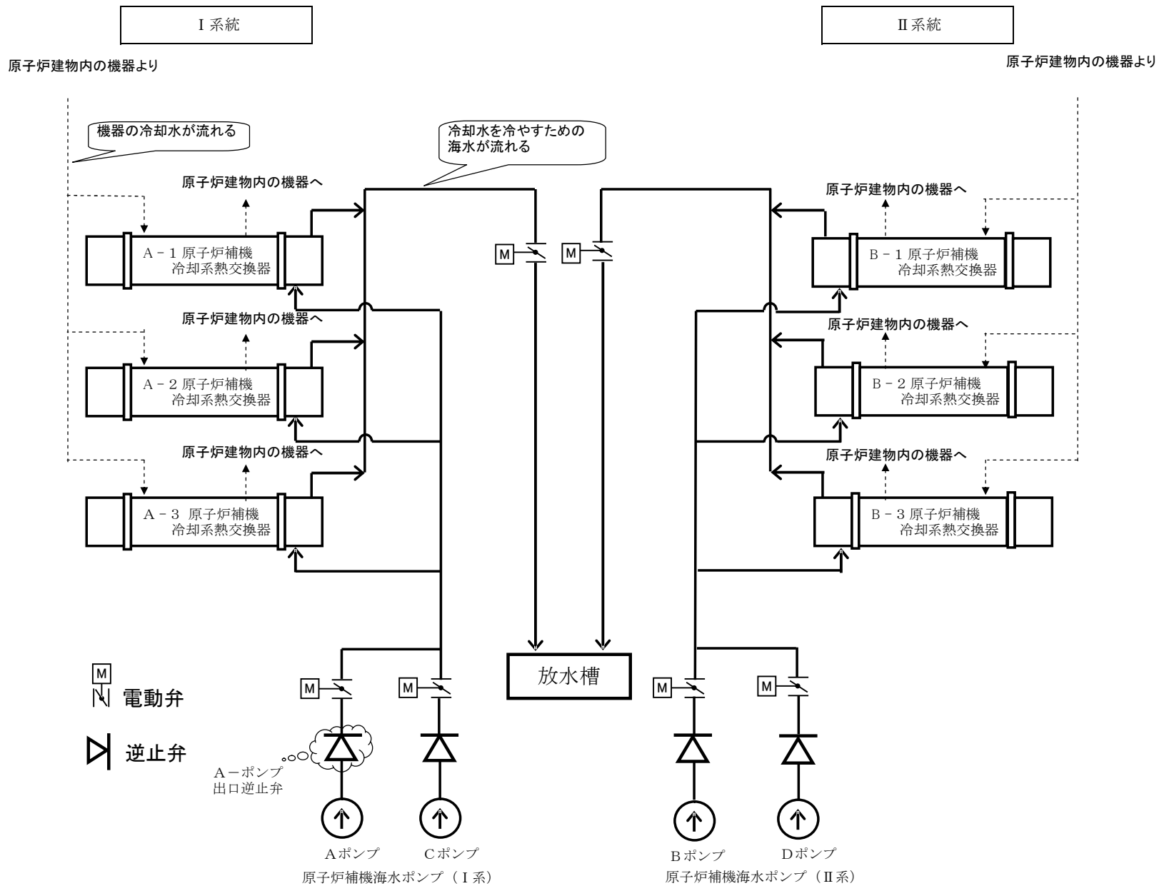
島根原子力発電所 2号機原子炉補機海水系系統図
