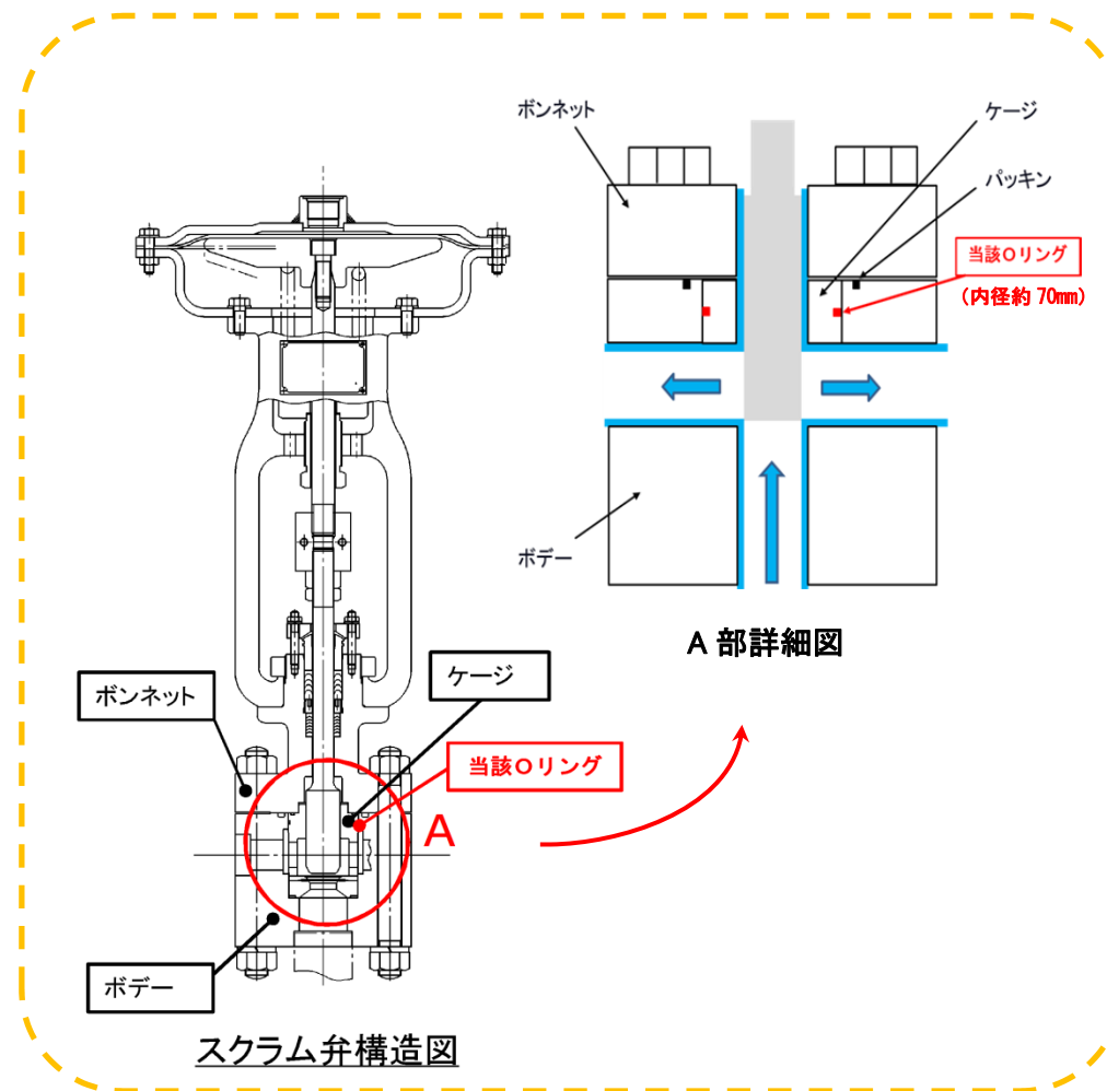
島根原子力発電所3号機 制御棒駆動系およびスクラム弁概要図
