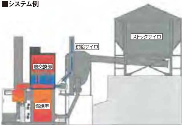
供給サイロを設置することで搬送トラブルをなくした。
