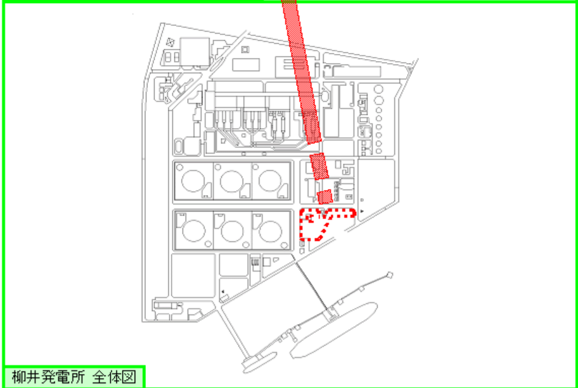
LNGローリー出荷設備 配置拡大図
