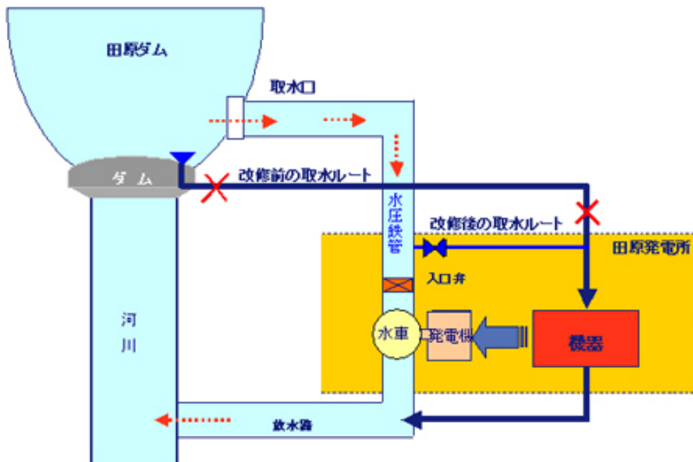
<田原発電所機器冷却用取水ルート図>
